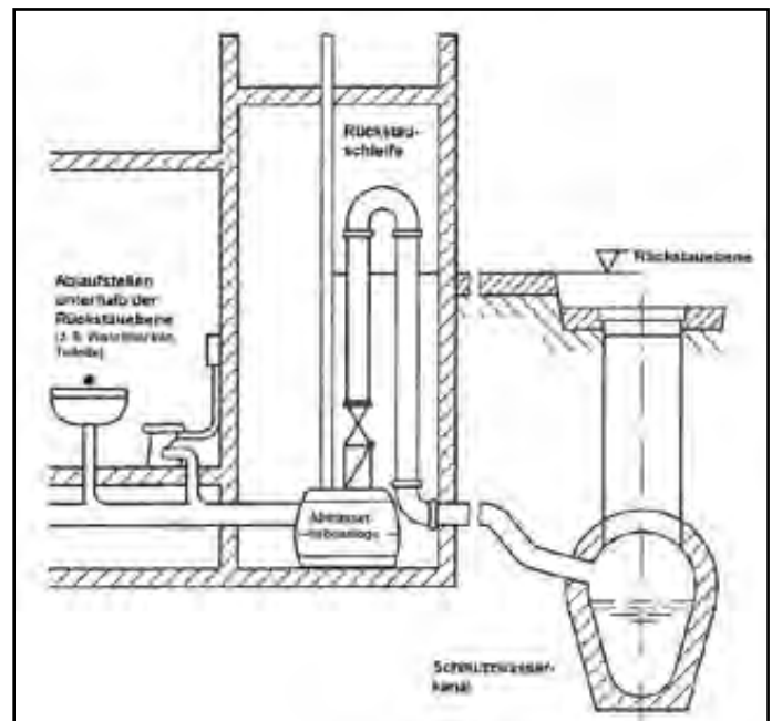
Abbildung 2: Prinzipskizze für den Einbau einer Abwasserhebeanlage zur Rückstausicherung
