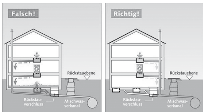
Abbildung 3: Einbau eines Rückstauverschlusses zur Sicherung von Fußbodenentwässerungen in Kellerräumen mit untergeordneter Bedeutung
